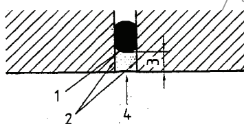
Σχήμα 3 - Απλή εξασφάλιση στεγάνωσης αρμού 1.Οπίσθια όψη του υλικού σφράγισης 2.Επιφάνεια επαφής του υλικού σφράγισης 3.Βάθος σφράγισης 4.Όψη του υλικού σφράγισης
