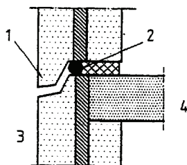
Σχήμα 4 - Διπλή εξασφάλιση στεγάνωσης αρμού σε προκατασκευασμένα στοιχεία όψεων (κάθετος τομή) 1.Διαμόρφωση της κατάληξης του κάτω άκρου υπό μορφή νεροστάλακη (πρώτη εξασφάλιση στεγάνωσης) 2.Υλικό σφράγισης (δεύτερη εξασφάλιση στεγάνωσης) 3.Έξω 4.Μέσα
